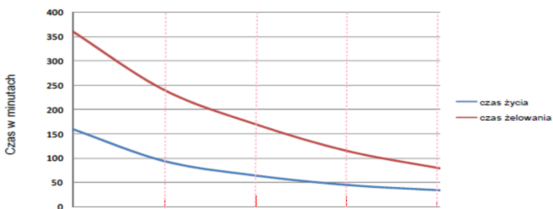
Zależność czasu życia oraz czasu żelowania od wzajemnej proporcji utwardzaczy EPOLAM 2017 oraz EPOLAM 2018 w 25°C
